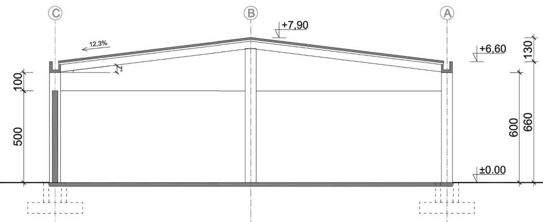
PRESJEK 1-1
